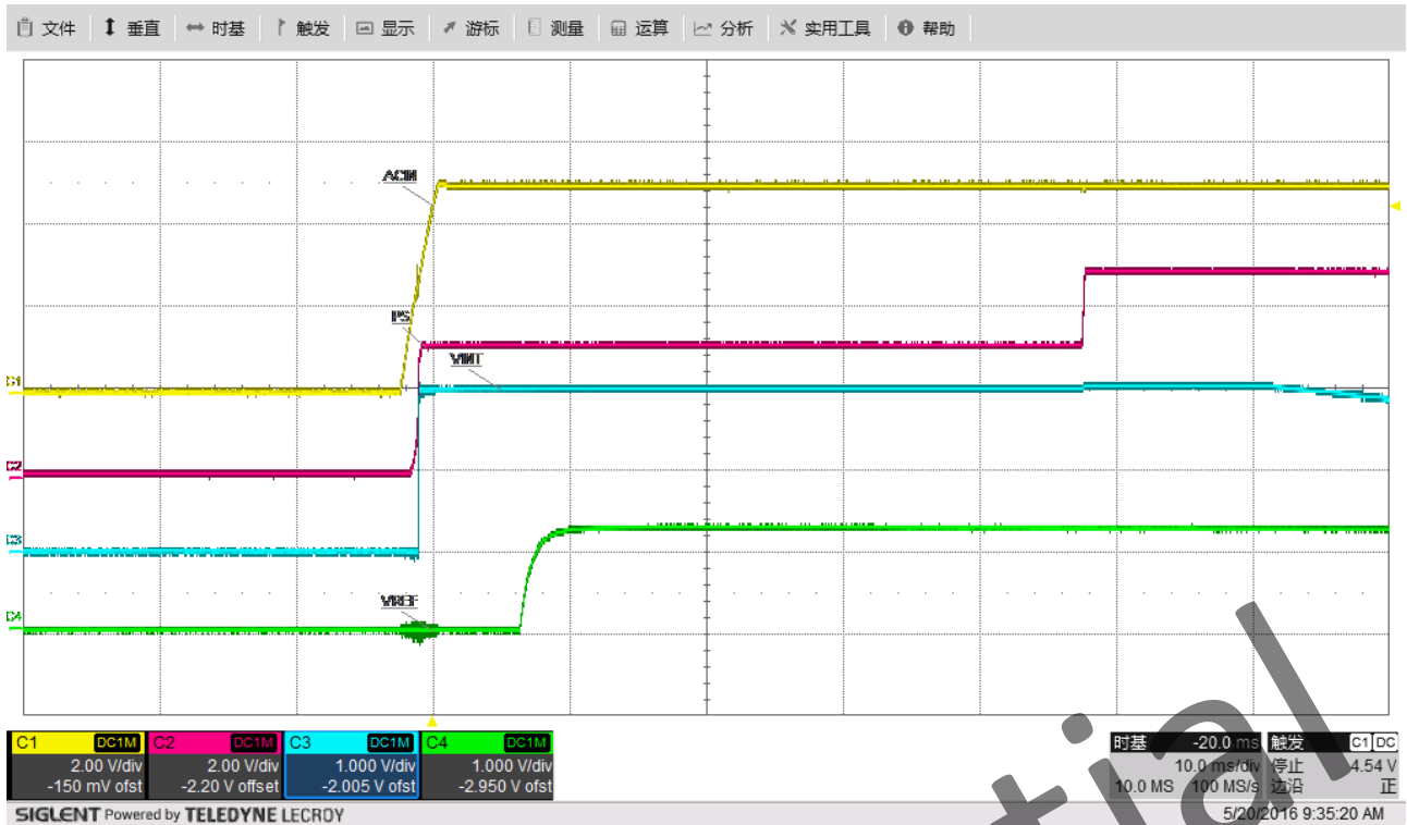
图 9.上电时序(ACP, PS, VINT, VREF)
