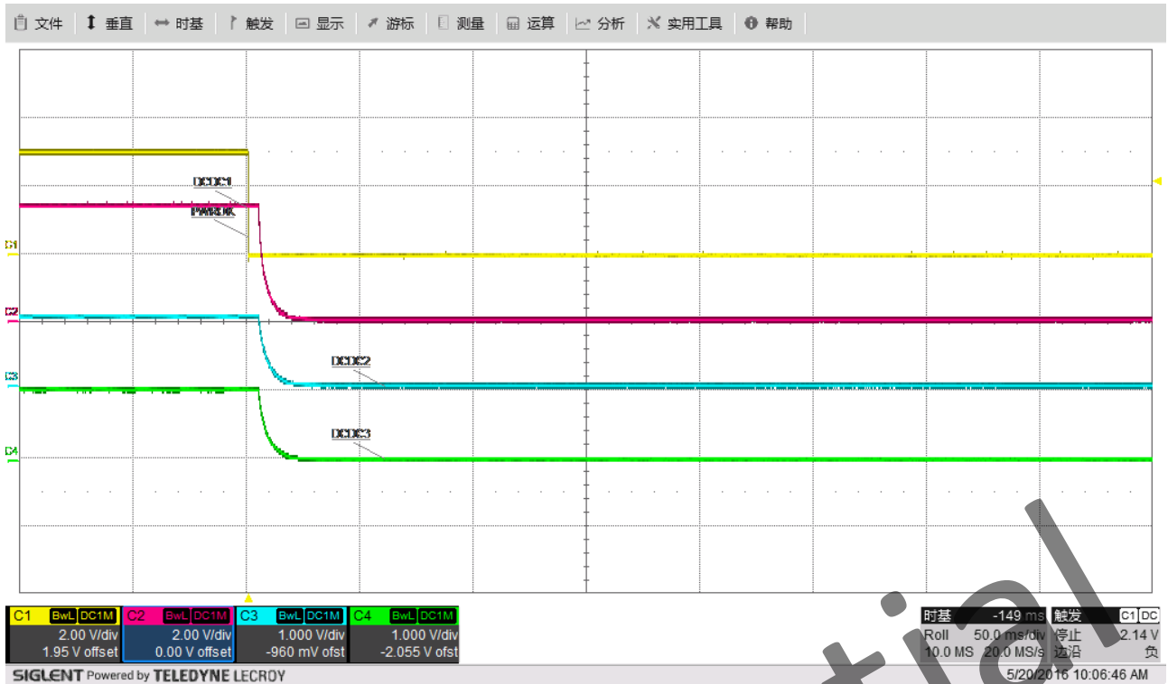
图 15.下电时序(PWROK, DCDC1, DCDC2, DCDC3)
