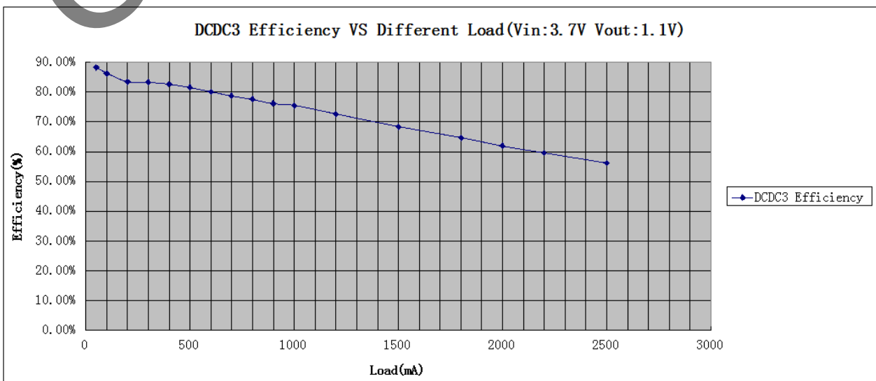
图 6. DCDC3 效率图 VS 负载
