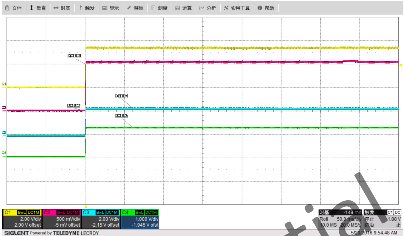
图 11.上电时序(DCDC1,DCDC3,DCDC4,DCDC5)
