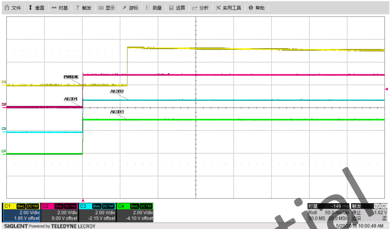
图 13.上电时序(PWROK, ALDO1, ALDO2, ALDO3)
