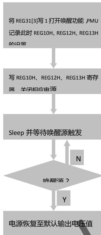
图 17. 休眠和唤醒控制流程
