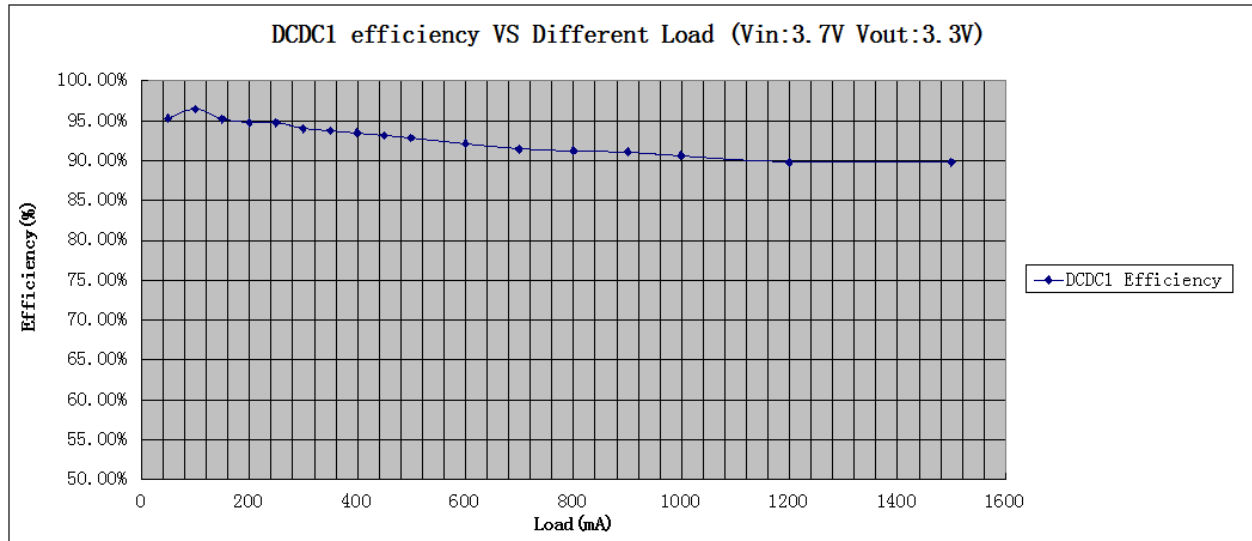
图 4. DCDC1 效率图 VS 负载
