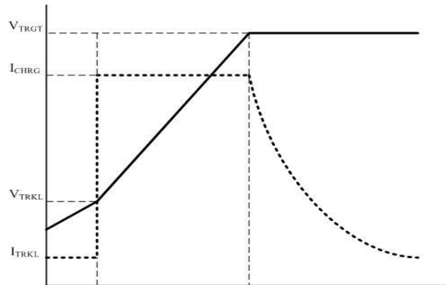
图 18. 充电电压电流示意图
