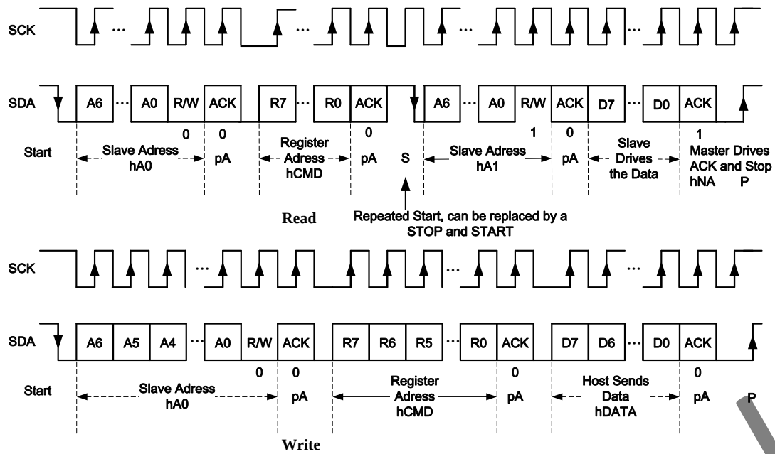
图 20 . TWSI 读写波形图
