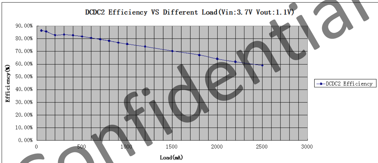
图 5. DCDC2 效率图 VS 负载
