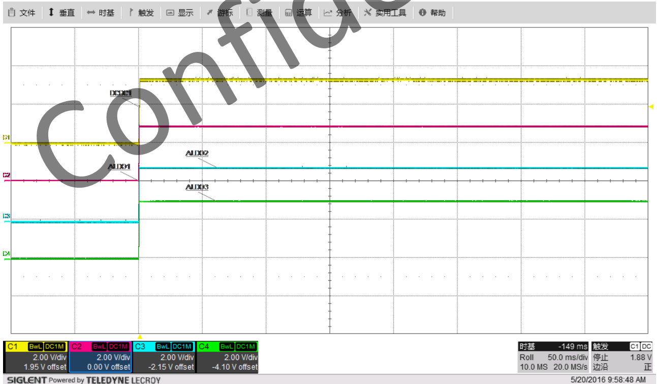
图 12.上电时序(DCDC1, ALDO1, ALDO2, ALDO3)
