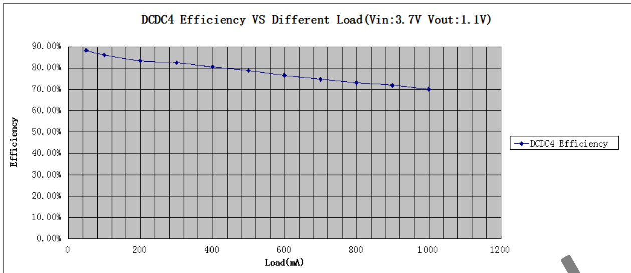
图 7. DCDC4 效率图 VS 负载
